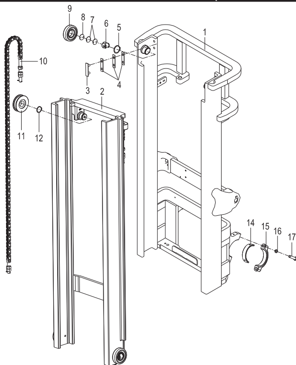
门架(基本型) /
