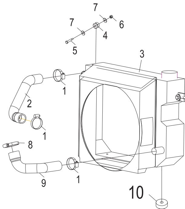
图6/FIG.6 冷却系统/Cooling system
