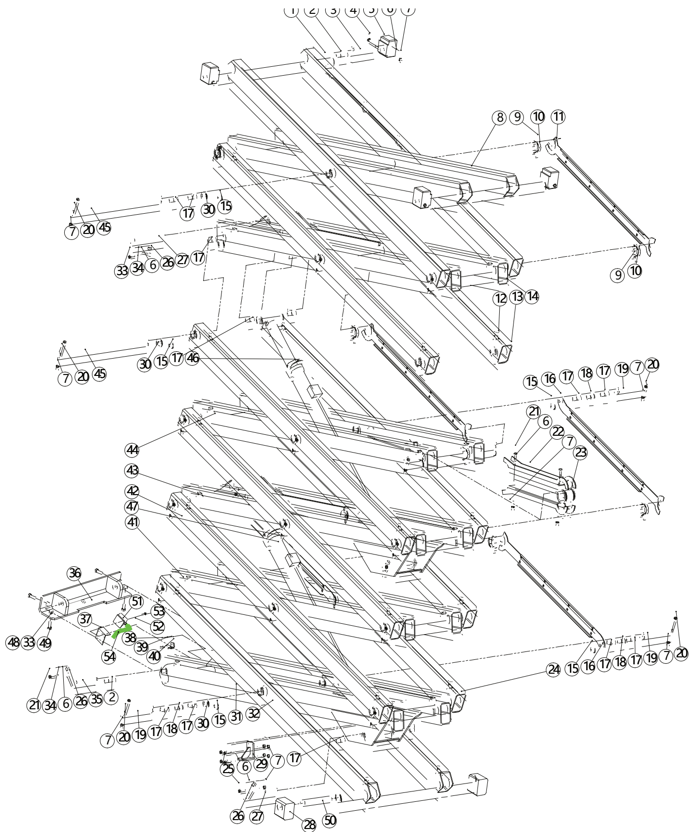
Figure 9 Pièces et composants des ciseaux(SC14H/SC14E)
