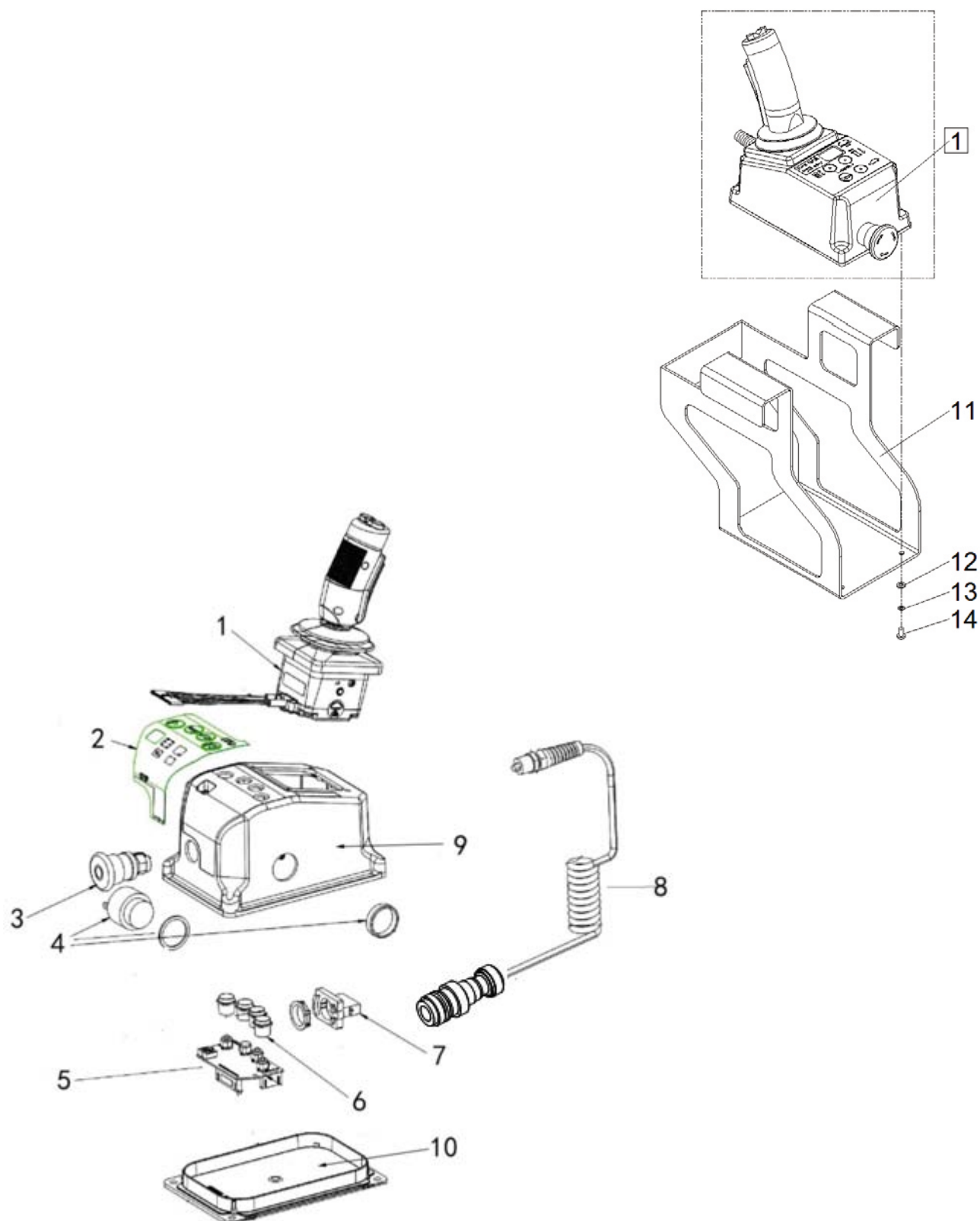
Figure 15 Composants du contrôleur de plateforme
